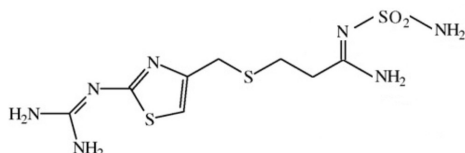
Figura 1. Estrutura química da famotidina
